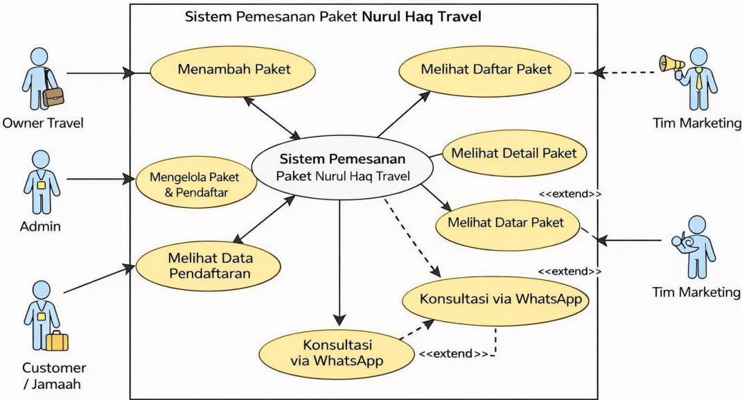
Use Case Diagram - Sistem Pemesanan Paket Nurul Haq Travel
